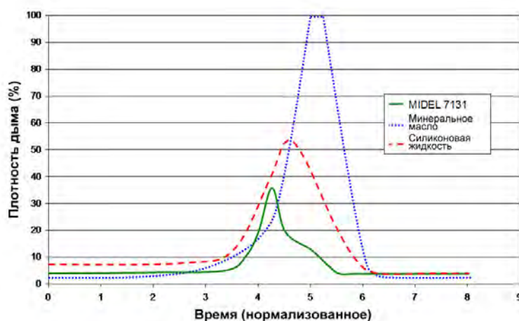
Рис. 2. Сравнение плотности дыма MIDEL 7131, силиконовой жидкости и минерального масла
