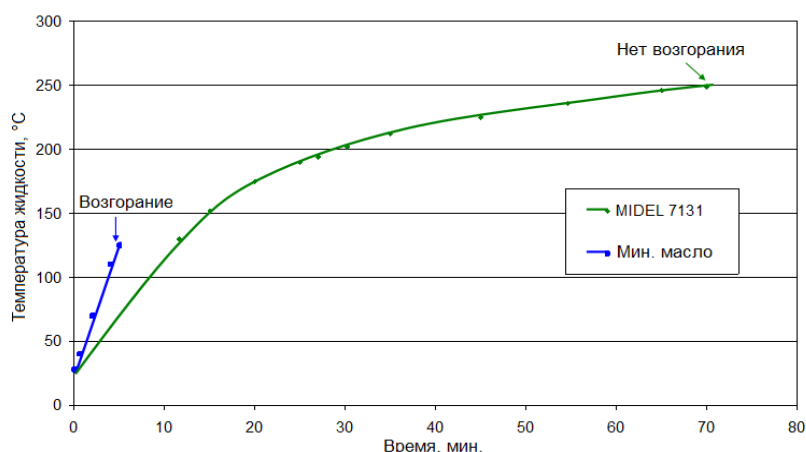
Рис. 1. Сравнение способности к возгоранию MIDEL 7131 и минерального масла
