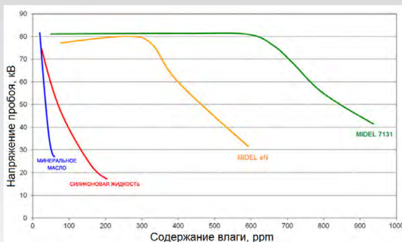
Рис. 8. Зависимость напряжения пробоя от содержания влаги при 20 °C
